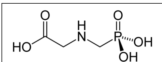
Figura 1: Formula di struttura del Glifosate
