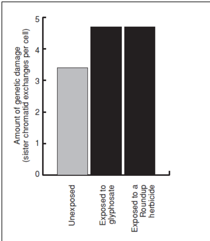
Figura 4: Differenze in campioni trattati e non trattati delle variazioni genetiche nelle cellule del sangue umano (tratto da Cox, 2994 su dati di Bolognesi et al. 1997)
