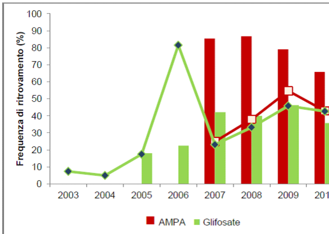
Figura 8: Frequenza di ritrovamento e di ricerca del Glifosate e dell'AMPA nelle acque superficiali. L'istogramma rappresenta la frequenza di ritrovamento e la curva descrive la frequenza di ricerca (ISPRA, 2013).
